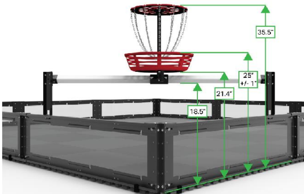
图 20 高筐的垂直尺寸
